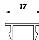
BX10-019 0,090kg/m
