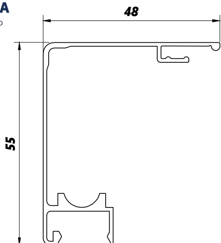
BX918 0,488kg/m
