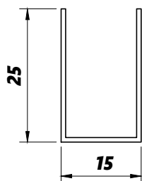
BX10-017 0,146kg/m
