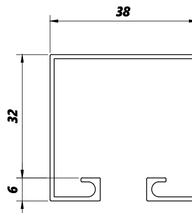
DS-314 0,450kg/m
