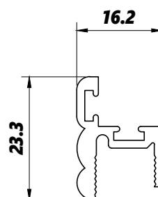
BX10-016 0,294kg/m
