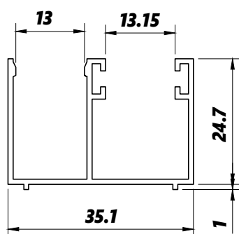
BX10-015 0,317kg/m
