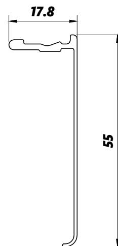
BXL913 0,211kg/m
