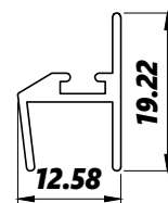
BX08-009 0,138kg/m
