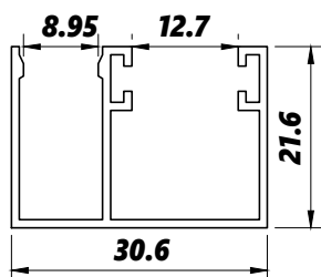
BX08-008 0,285kg/m
