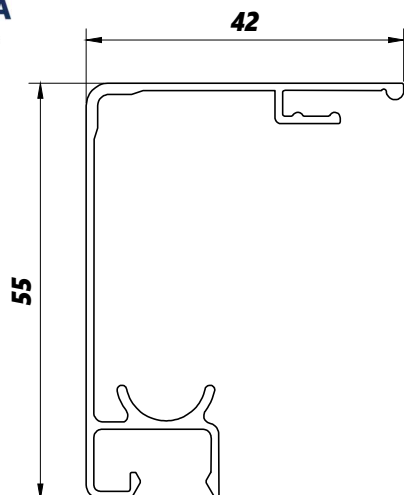
BX919 0,451kg/m
