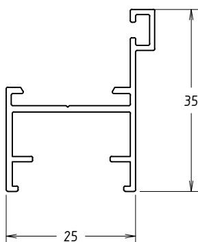
SU079 0,307kg/m
