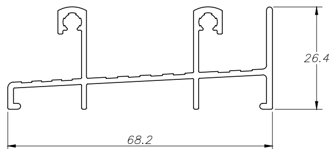
SU260 0,674kg/m
