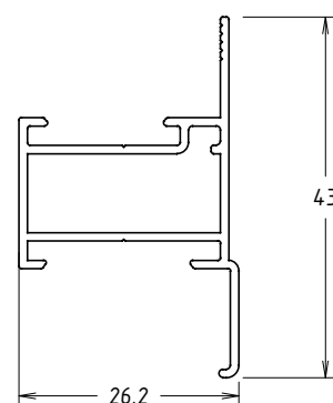
SU081 0,331kg/m
