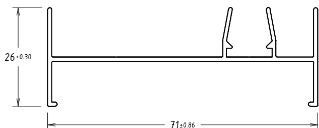
SU003 0,465kg/m
