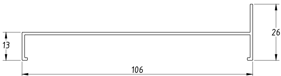
SU012 0,471kg/m
