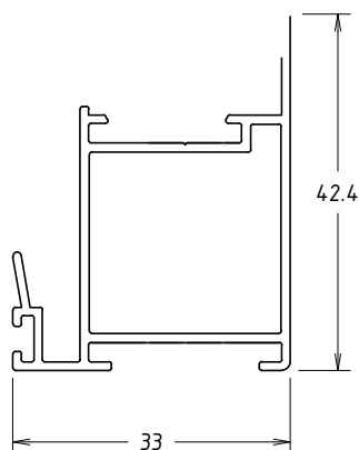
SU041 0,453kg/m
