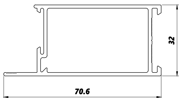
ALG043 0,830kg/m
