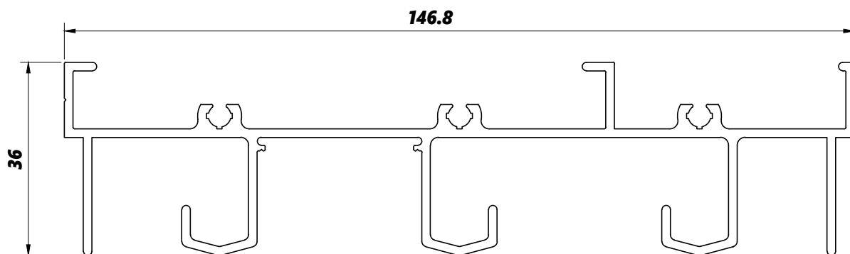
LG062 1,728kg/m
