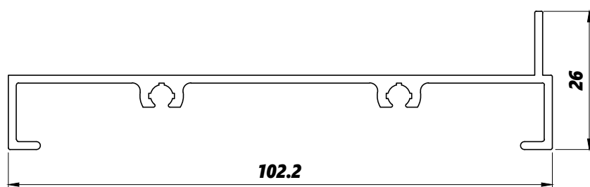
LG003 0,756kg/m
