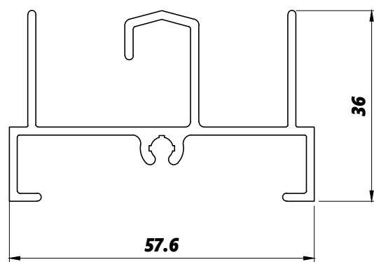
SL348 0,790kg/m
