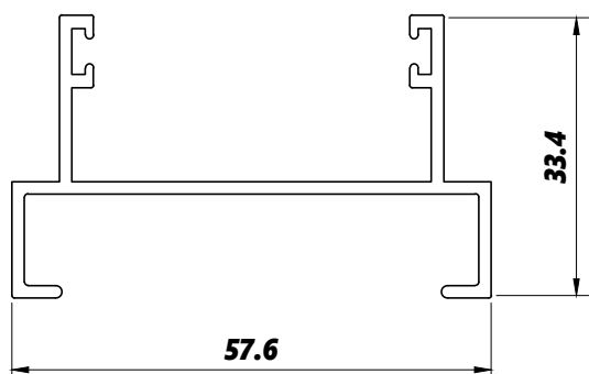
SL349 0,591kg/m
