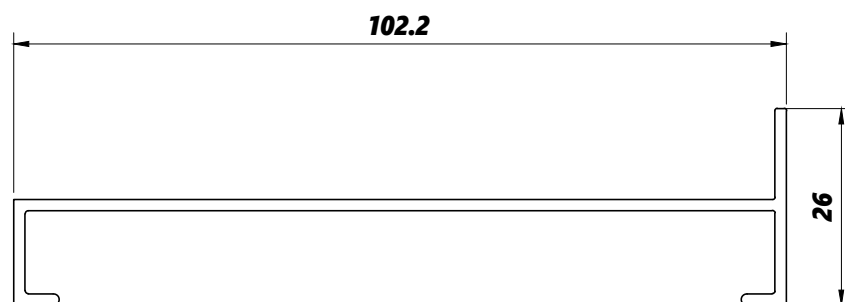
LG002 0,601kg/m
