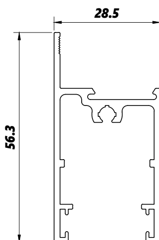
LG006 0,676kg/m
