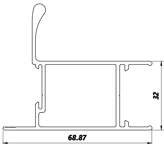
LG017 1,008kg/m
