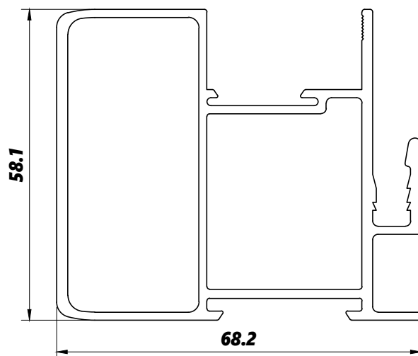
LG018 1,570kg/m
