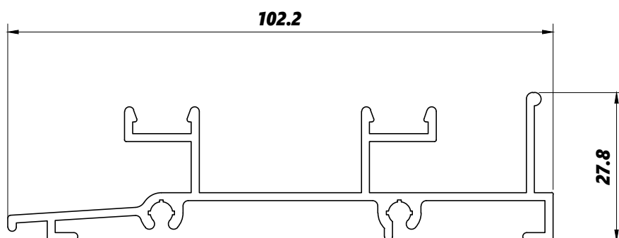
LG125 0,991kg/m
